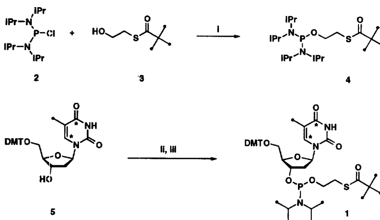
Scheme 1 I: EtN(iPr) 2 /CH 2 Cl 2 ; ii: 1 H -tetrazole/MeCN/CH 2 Cl 2 ; iii: aq NaHCO 3 .
